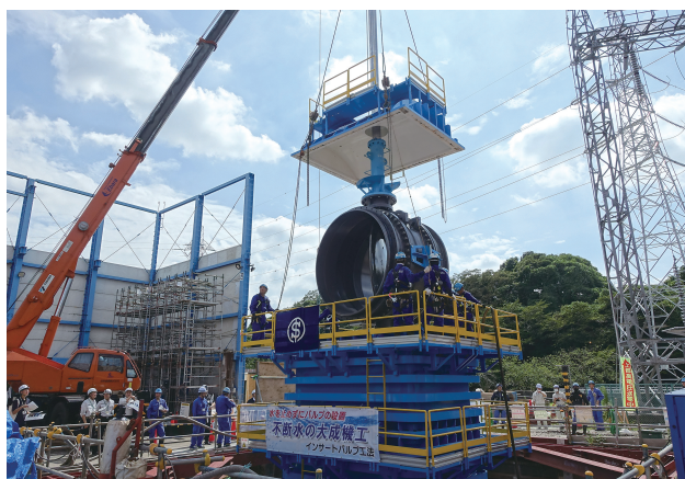
7月17日に世界最大となるφ2400バタフライ弁をインサート工法で施工(北千葉浄水場内)
